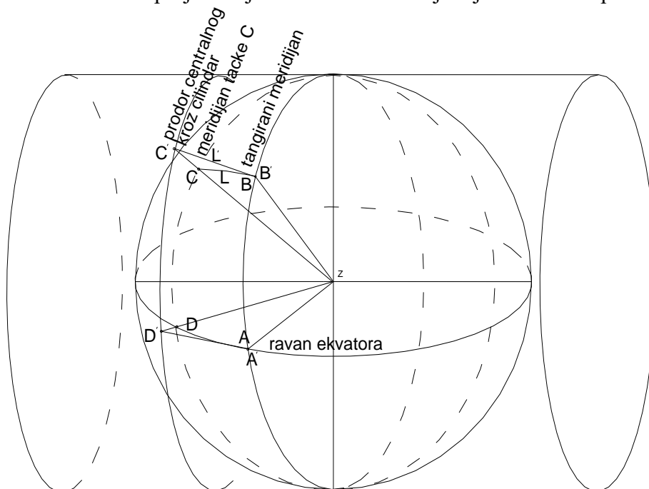
Slika 3. Gaus – Krigerova projekcija – projekciranje linija
