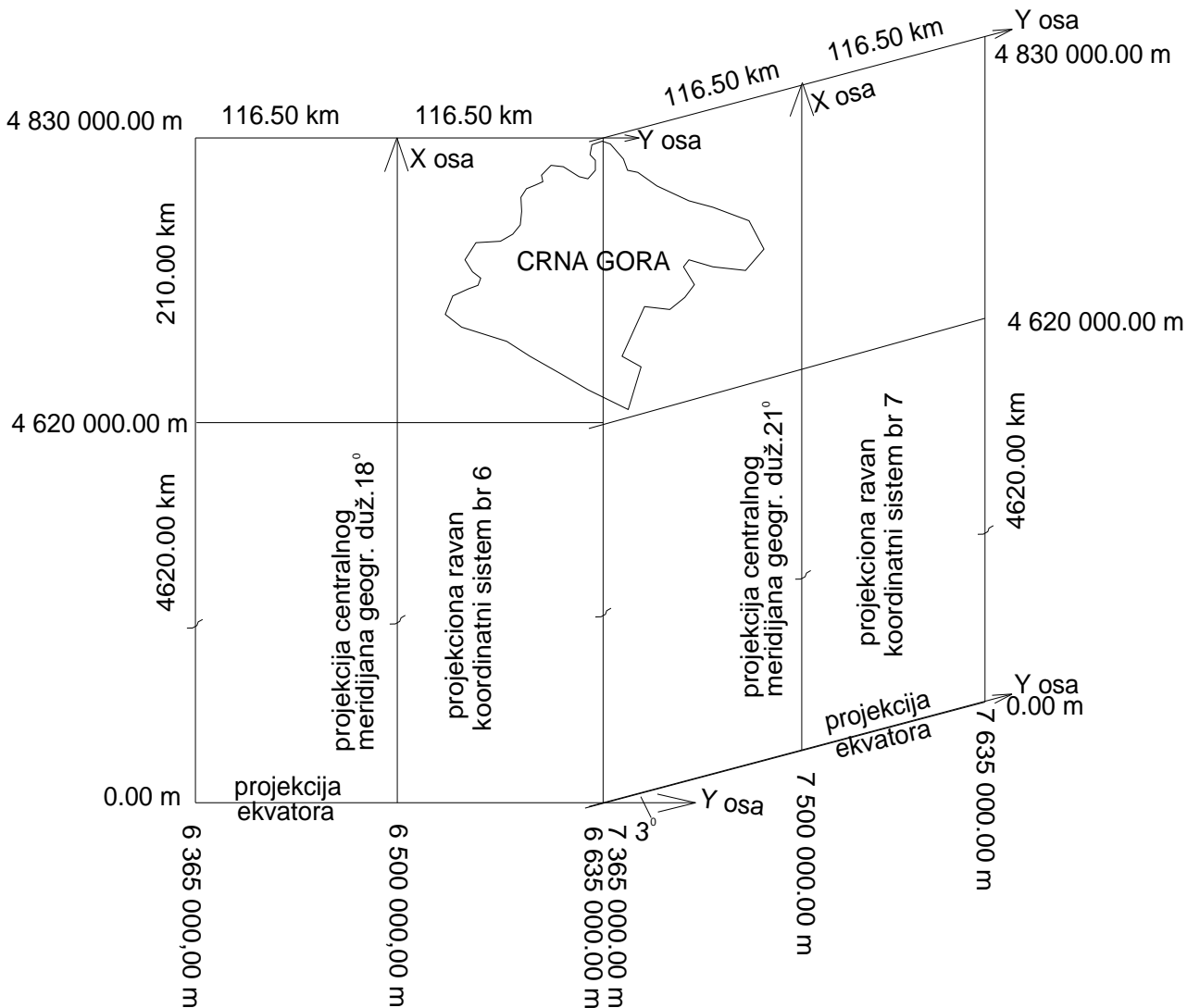
Slika 6. Projekcione ravni 6 i 7
