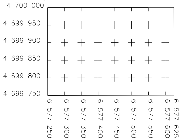
Slika 16. Decimetarska mreža na listu R 1:500
